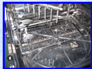
ポリ容器洗浄治具 (オプション)
